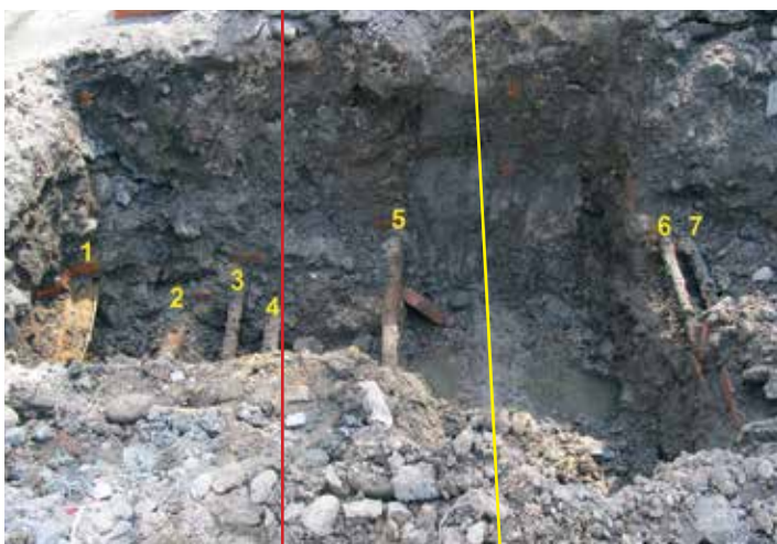
Ulica Stroma. Według map geodezyjnych w tym miejscu powinny znajdować się tylko dwa kable (nr 2 i 5), a jest ich łącznie 7. Czerwona linia - planowany przebieg budowanej kanalizacji. Żółta linia - istniejący kanał ogólnospławny.
